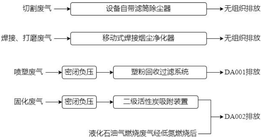
图 4-1 废气收集、处理走向图
