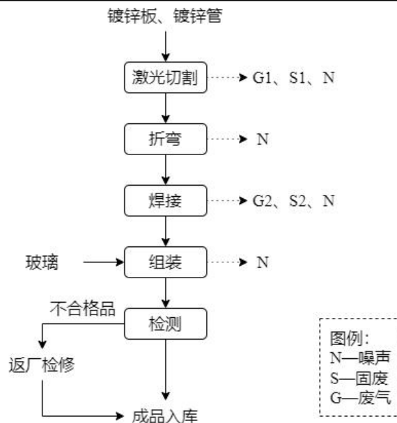
图 2-3 现有项目工艺流程图
