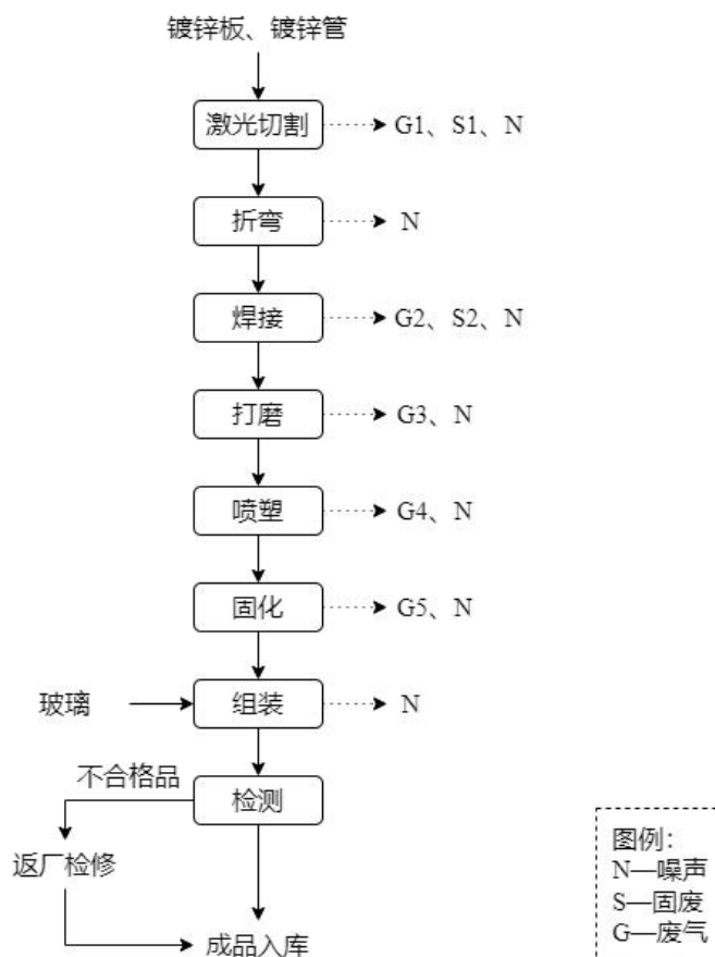
图 2-2 工艺流程图
