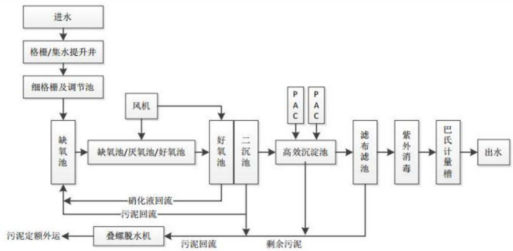
图 4-2 关庙镇污水处理厂工艺流程图
